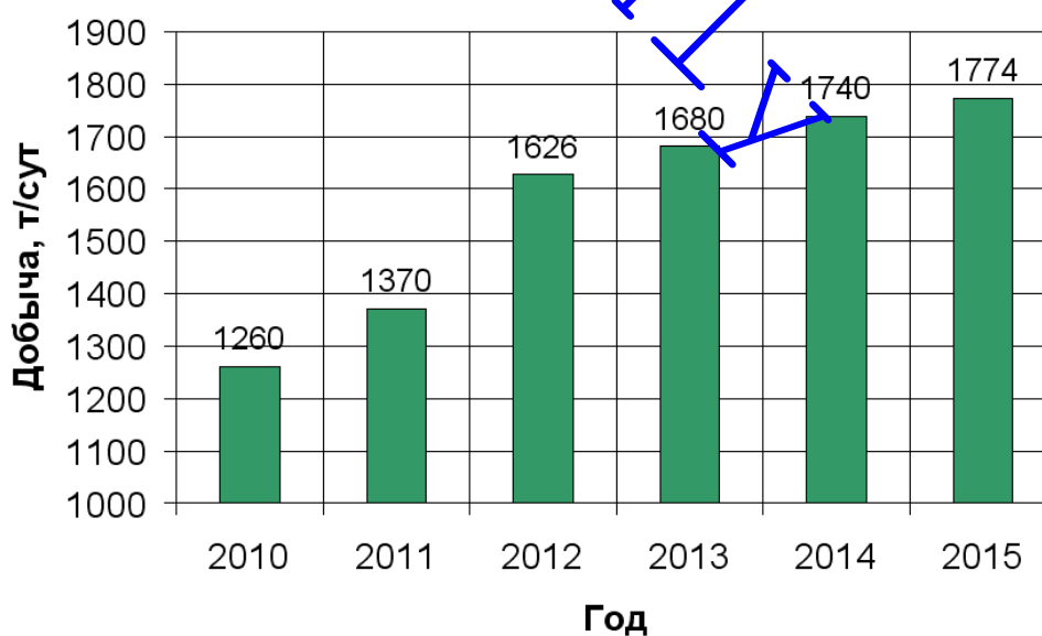
Рисунок 1.1 – Среднесуточная добыча угля из лавы
