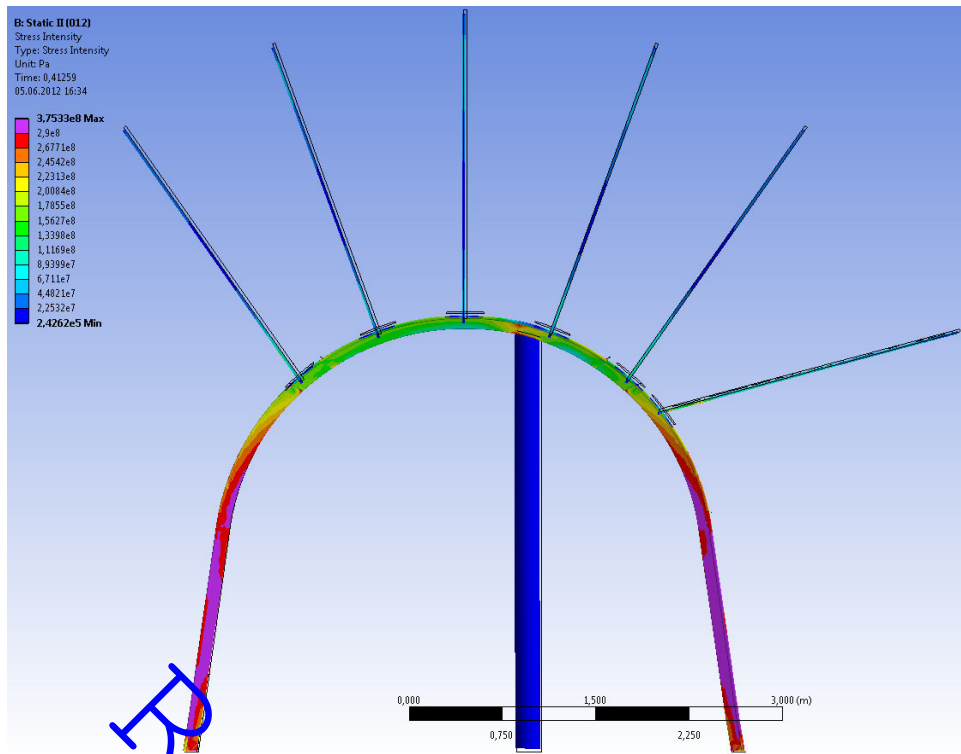
Рисунок 2.5 – Эпюра интенсивности напряжений \sigma в базовой крепежной системе выемочной выработки в начале зоны опорного давления
