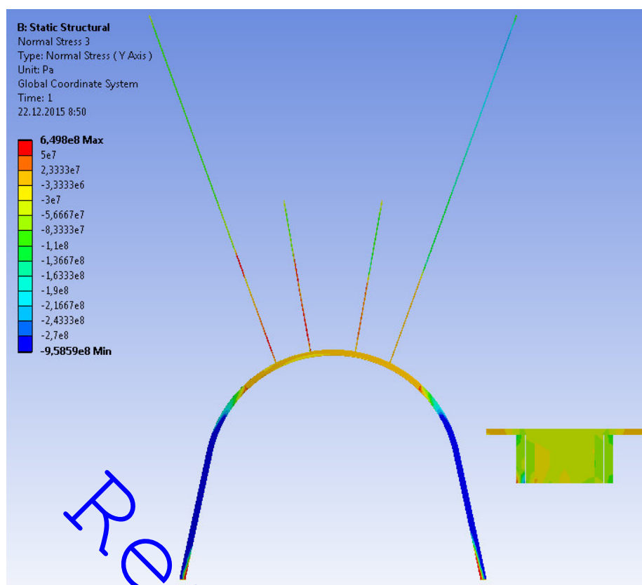
Рисунок 3.6 – Эпюры вертикальных напряжений \sigma_y в крепежных элементах выемочной выработки при использовании комбинированной анкерной системы
